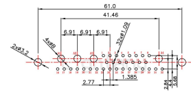
PCB布局 (PCB Layout)
